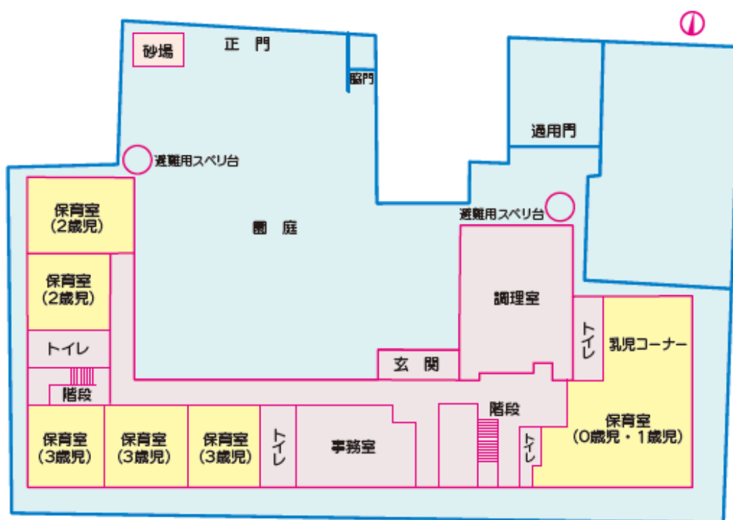
1階見取り図
